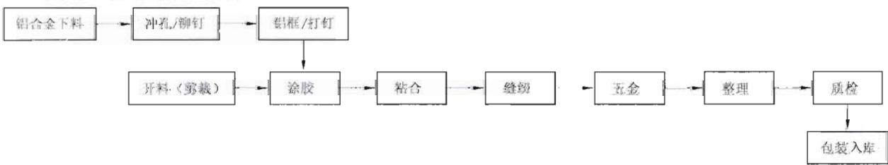
图 2 线缝箱包工艺流程图
